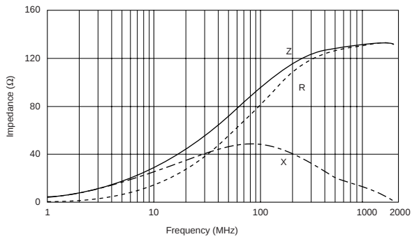
BLM18EG101TN1
