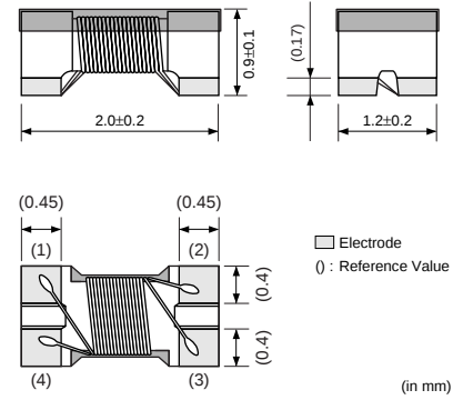
DLW21H系列
