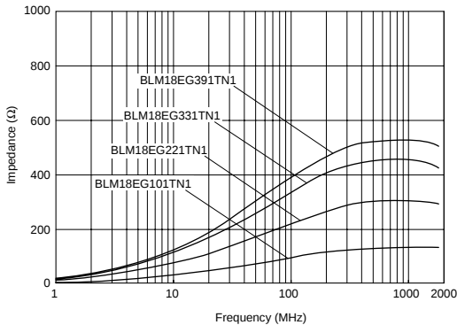
BLM18EG_TN系列
