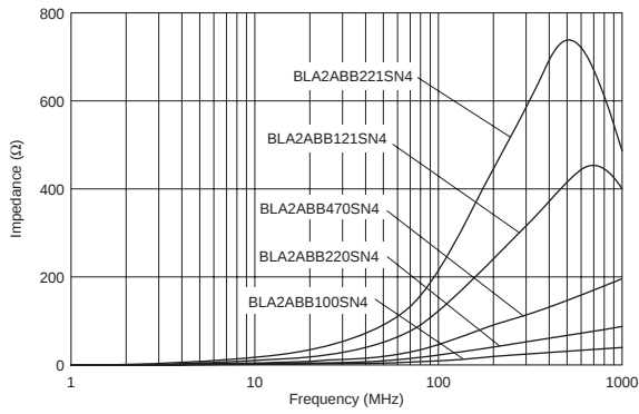
BLA2ABB系列
