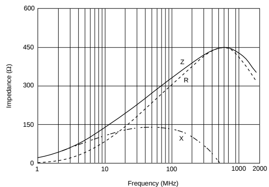
BLM18HK331SN1
