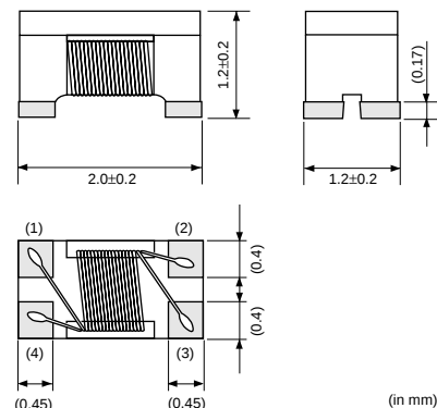
DLW21S_HQ系列
