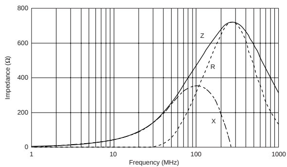
BLA2ABD471SN4
