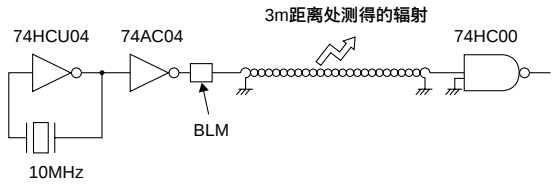
测试电路
