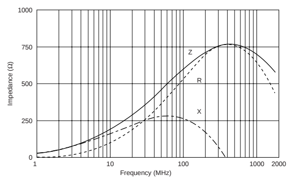
BLM18EG601SN1
