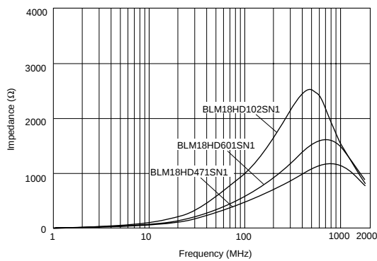
BLM18HD系列
