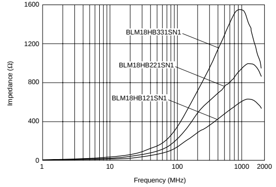
BLM18HB系列
