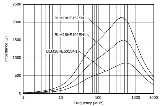
BLM18HE系列
