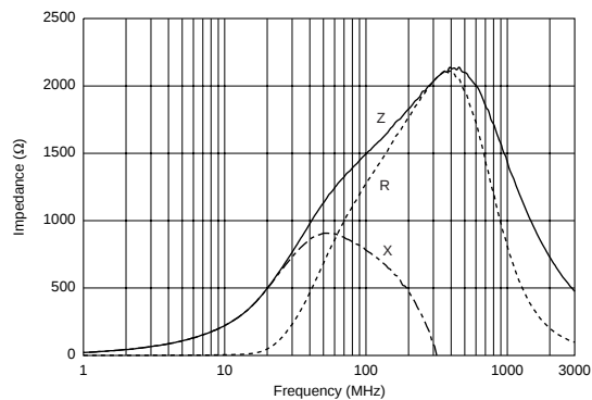
BLM18HE152SN1
