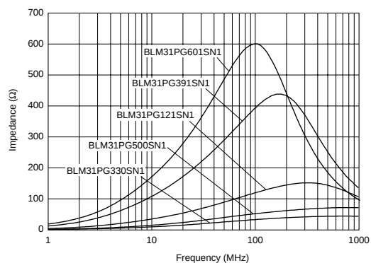
BLM31P系列
