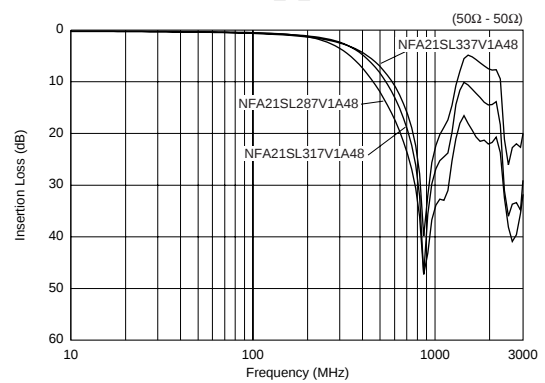
NFA21SL_V_48系列
