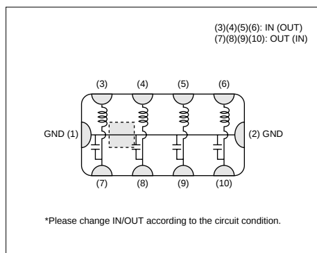
NFA18SL 137/187/207 V1A45
