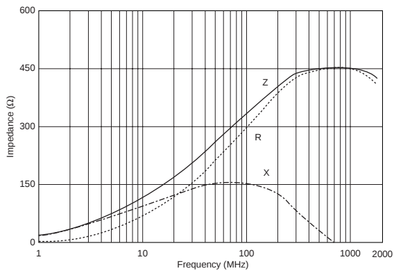
BLM18EG331TN1
