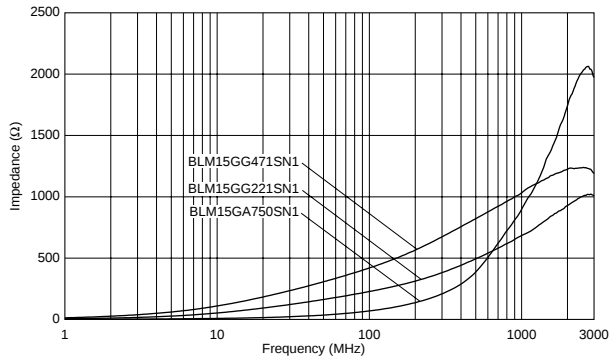
BLM15G系列
