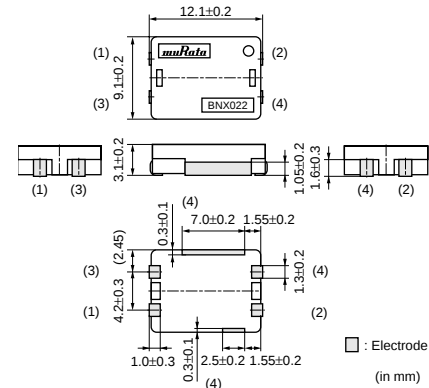
BNX022/023
