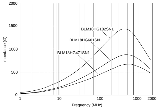
BLM18HG系列
