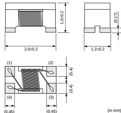
DLW21S_SQ系列
