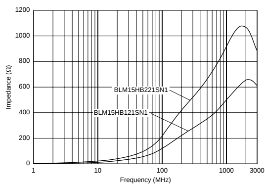
BLM15HB系列
