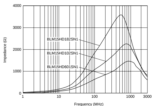
BLM15HD系列
