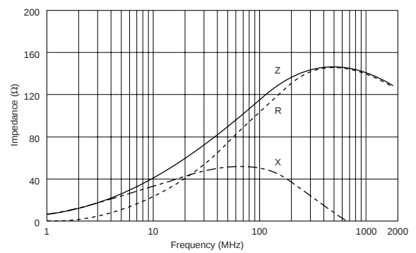
BLM18EG121SN1
