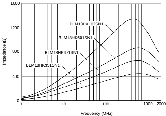
BLM18HK系列
