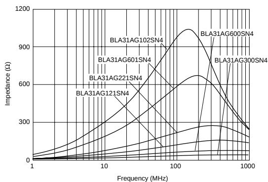
BLA31A系列
