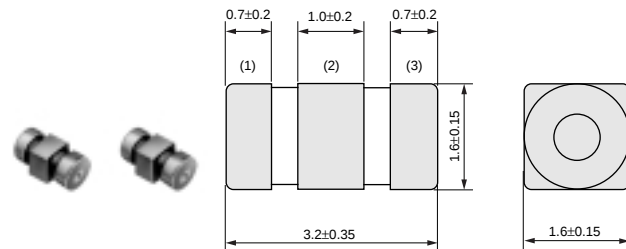
NFE31P系列
