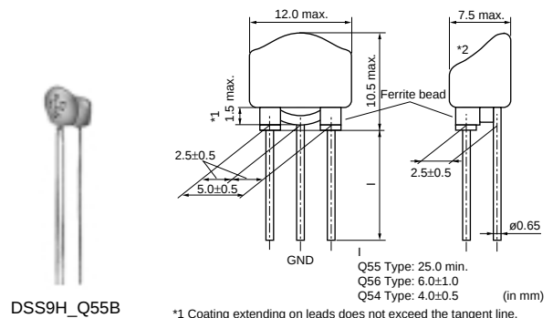
DSS9H_Q55B
