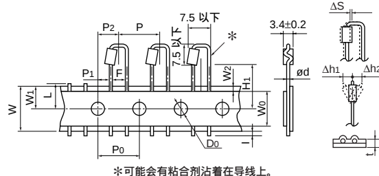
BL02RN2R1□1A
