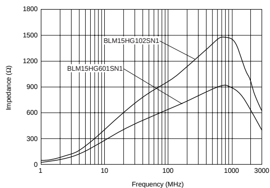
BLM15HG系列
