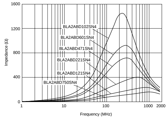
BLA2ABD系列
