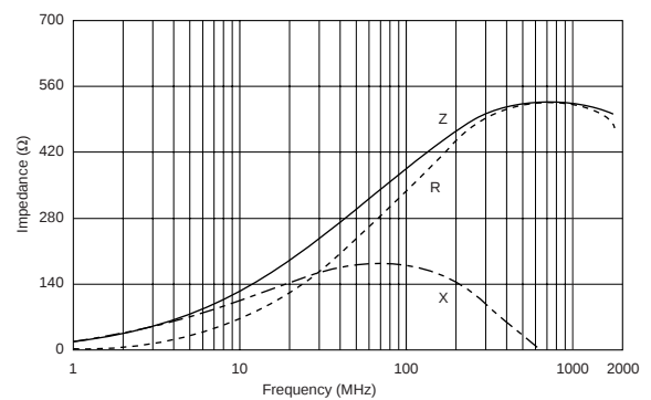
BLM18EG391TN1
