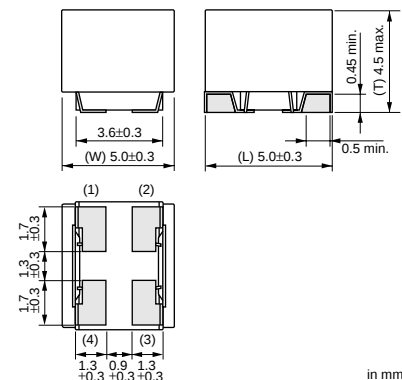
DLW5BS系列
