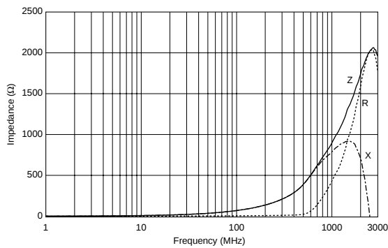
BLM15GA750SN1
