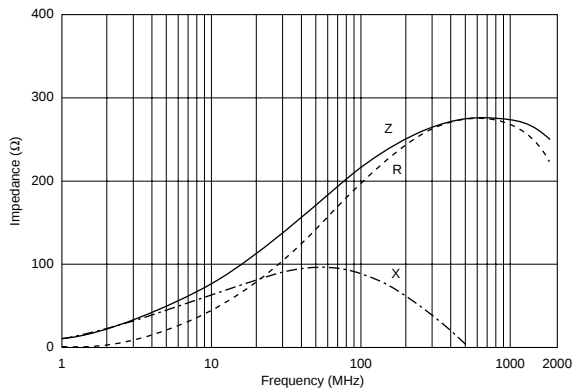
BLM18EG221SN1
