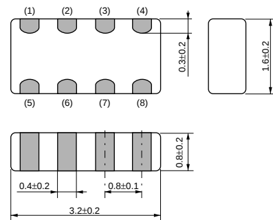
BLA31A/BLA31B系列
