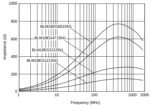
BLM18EG_SN系列
