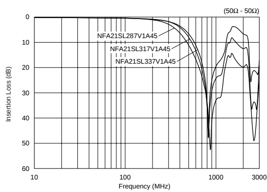
NFA21SL_V_45系列
