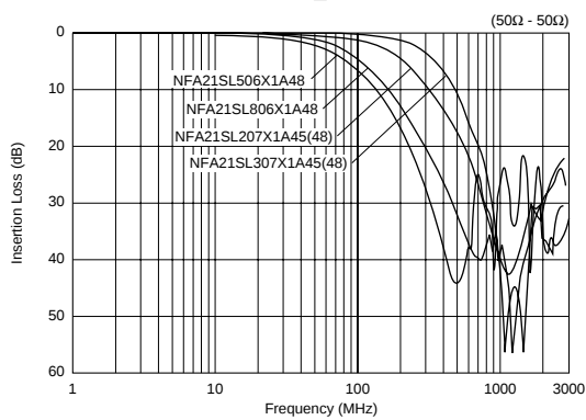
NFA21SL_X系列
