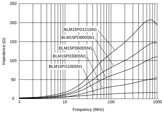
BLM15P系列
